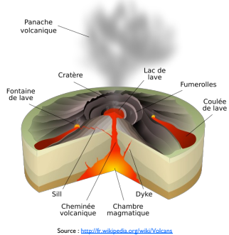
Source : http://fr.wikipedia.org/wiki/Volcan
