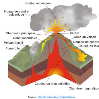
Source : http://fr.wikipedia.org/wiki/Volcan
